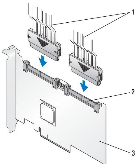
Рис. 4-2. Подсоединение кабелей
